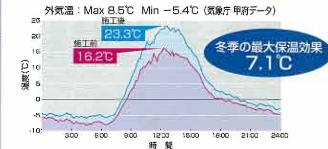
図-3 施工前後の冬季屋根表面温度変化 「ルーフェード」施工前(12/22)赤・施工後(12/22)青の温度変化
