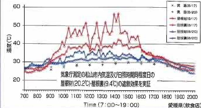
図-1 施工前後の屋根材・屋根裏の温度変化 「ルーフェード」施工前(8/17)赤・施工後(8/20)青の温度変化
